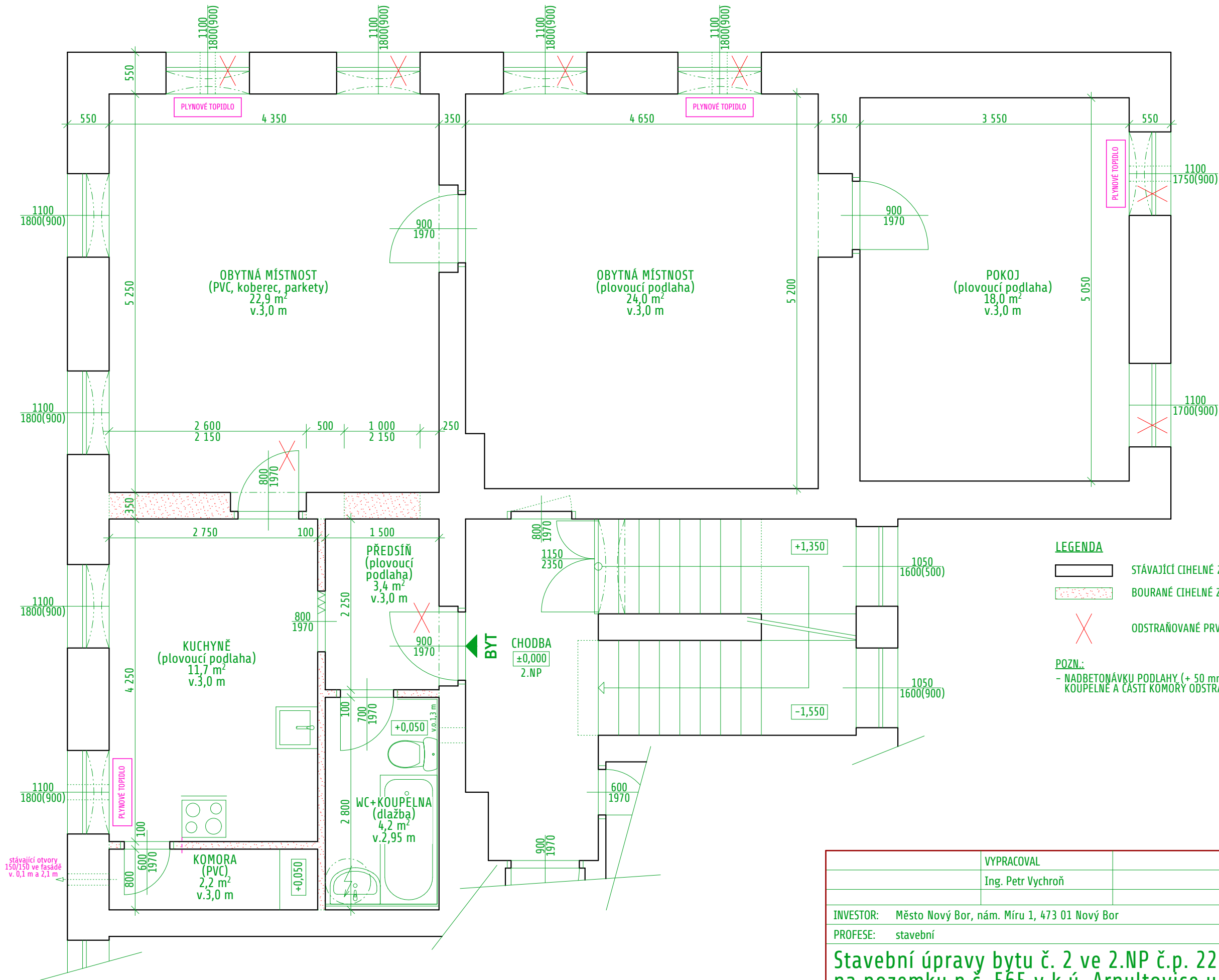
PŮDORYS 2.NP (byt č. 2) - STÁVAJÍCÍ STAV
