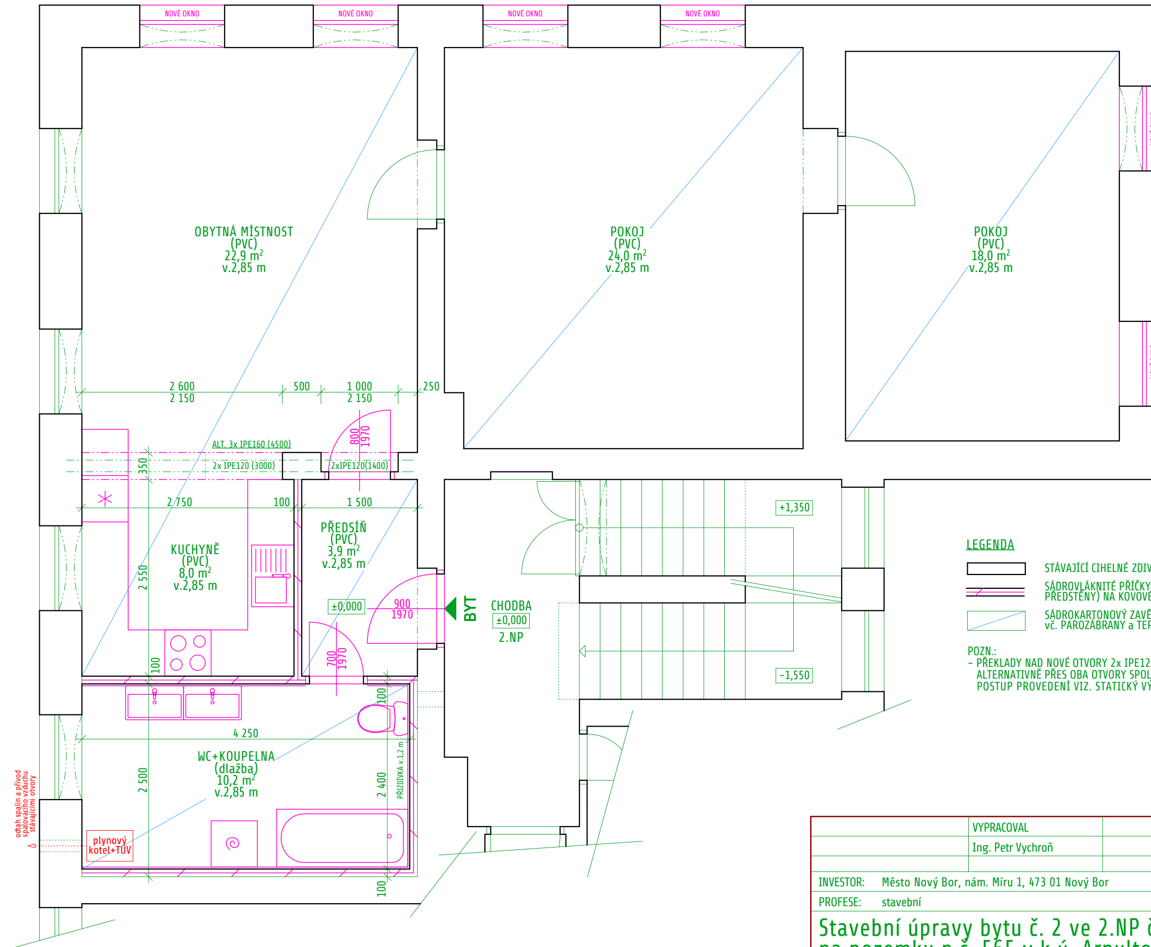
PŮDORYS 2.NP (byt č. 2) - NAVRHOVANÝ STAV
